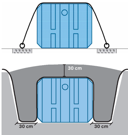
Exempel på förankring med hjälp av fiberduk (den svarta linjen) som i likhet med bilden läggs över tank och schakt innan återfyllning görs.
